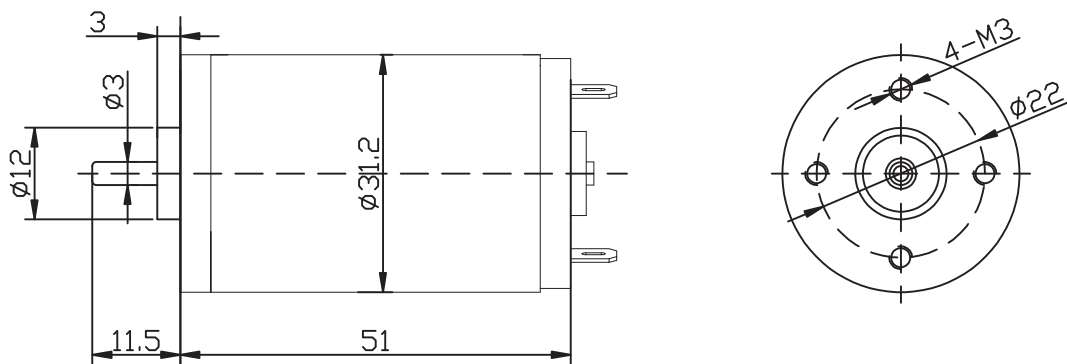
外形尺寸图/Appearance size
